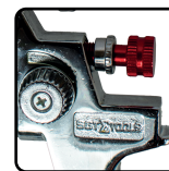
Regulagem de fluido, leque e ar separados. Permite ajustes finos e precisos
