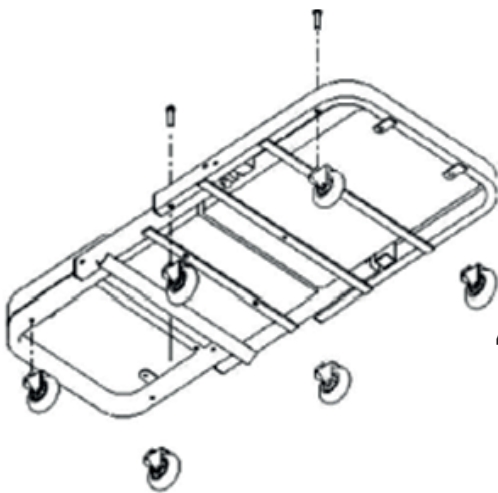
Figura 3 - Anexando os rodízios na estrutura
