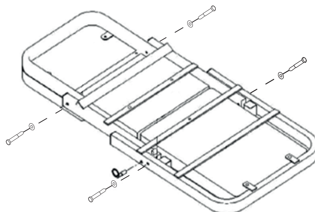
Figura 2 - Conjunto da seções da estrutura
