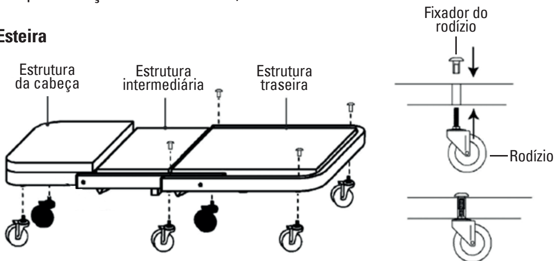
Figura 2 - Conjunto da seções da estrutura
