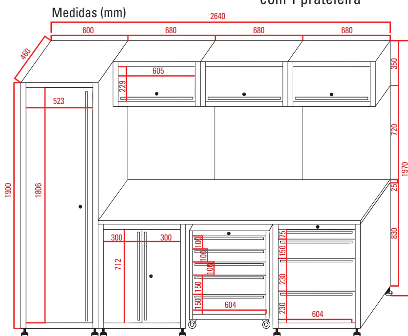
Armário inferior com 1 prateleira
